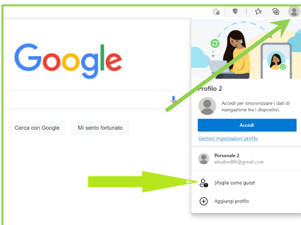
MICROSOFT EDGE
